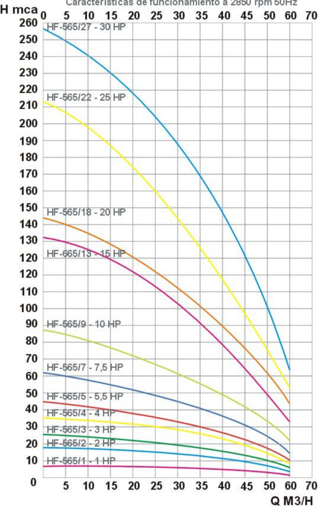
Características de funcionamiento a 2850 rpm 50Hz
