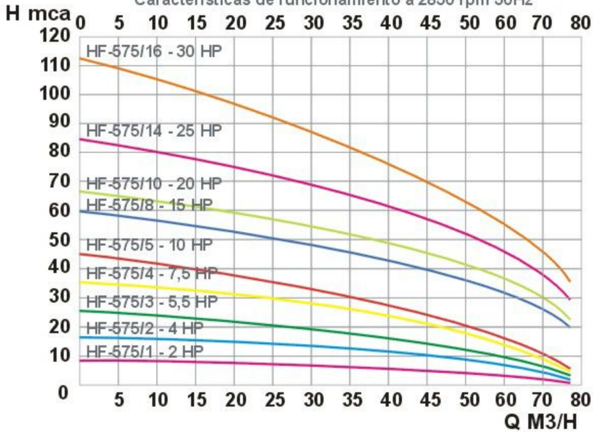
Características de funcionamiento a 2850 rpm 50Hz
